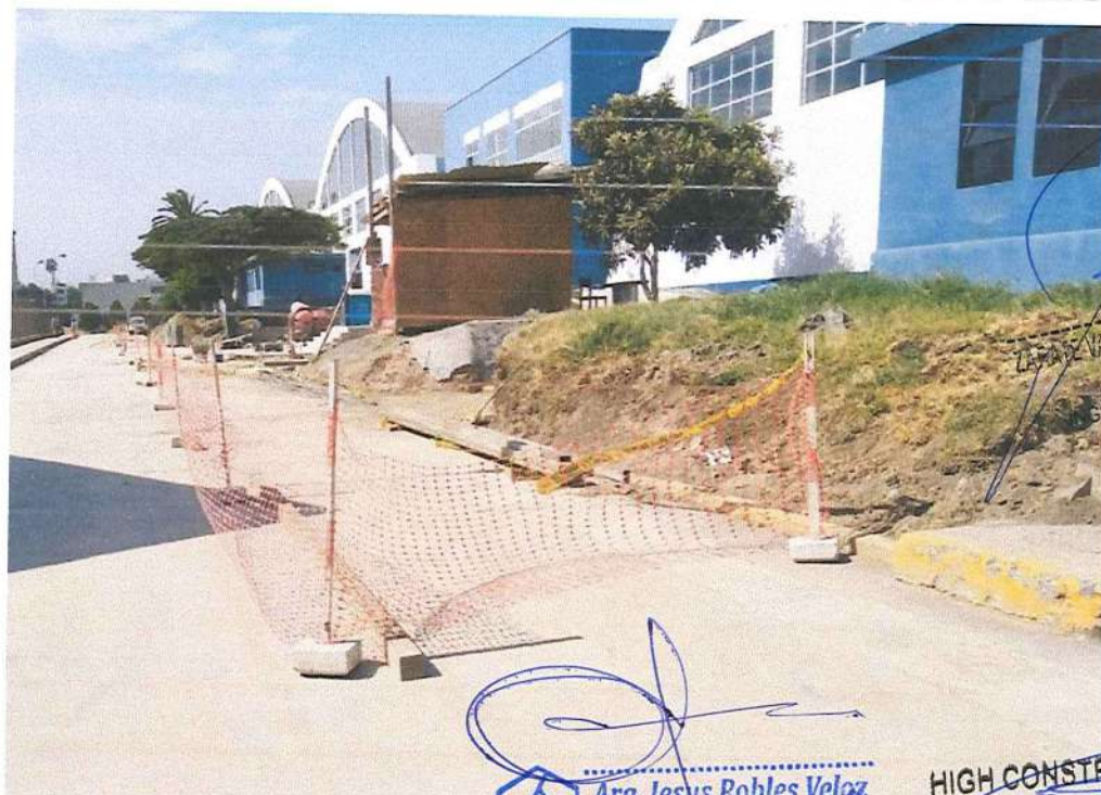
IMAGEN N°04: SEÑALIZACIÓN DEL ÁREA DE TRABAJO EN OBRA
