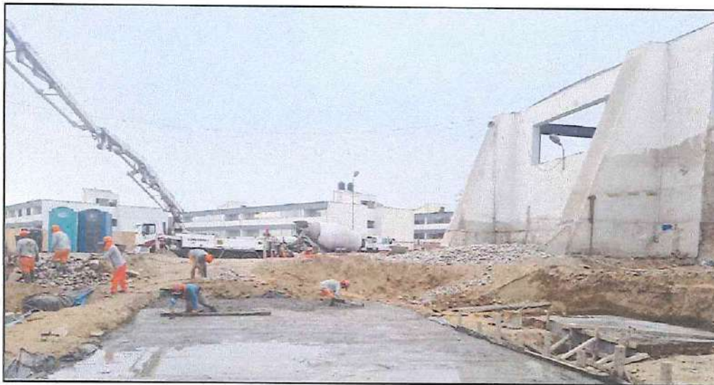
Imagen N° 23: Vaciado de concreto para falsa zapata
